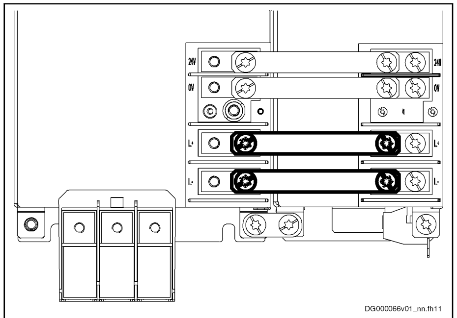
插图 5-7: 带连接排的直流母线连接
