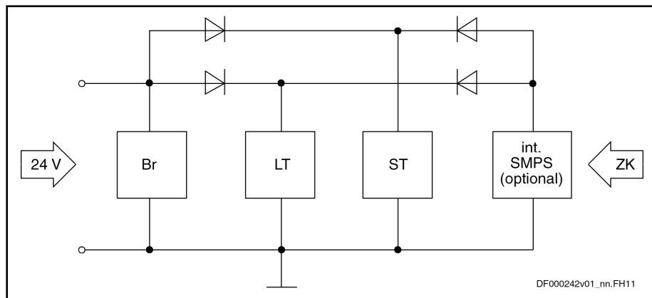
BR 制动控制电路 LT 功率部分，例如 HCS02 ST 控制装置，例如 CSB01 整型 SMPS 用于 HCS0x.1E-Wxxxx-NxxV 型号：内部切换模式电源 ZK DC 母线 插图 5-3: 内部控制电压框图
