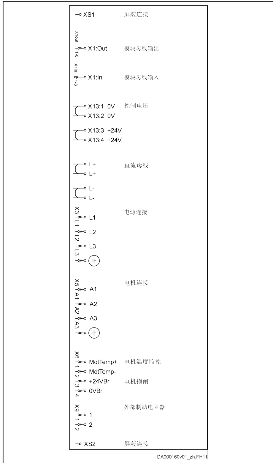
X1, L+/L- 对 HCS02.1E-W0012 不可用 X9 对 HCS02.1E-W0012 和 -W0028 不可用 插图 5-2: 总体连接图
