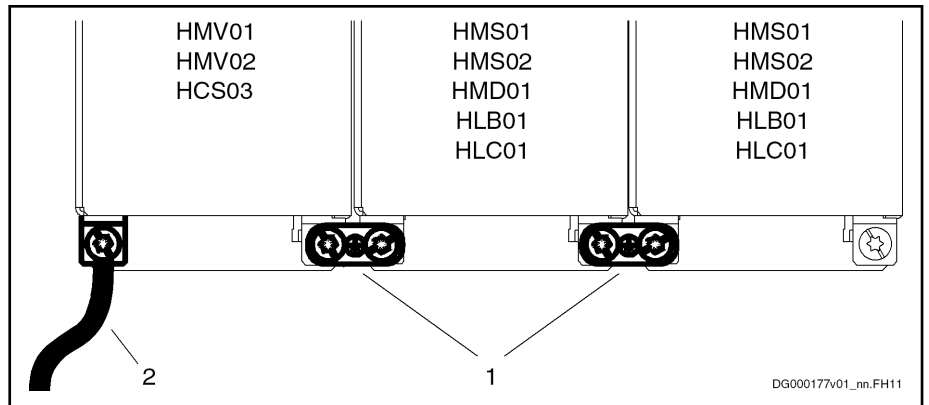
插图 5-7: 通过 HMV01、HMV02 和 HCS03 将设备接地导线连接到供电装置
