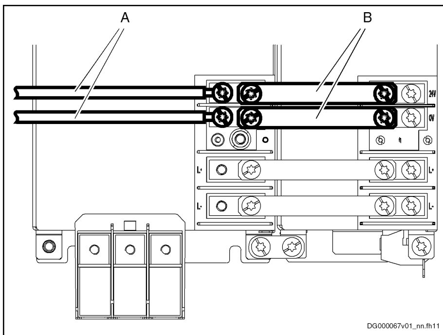
连接图
