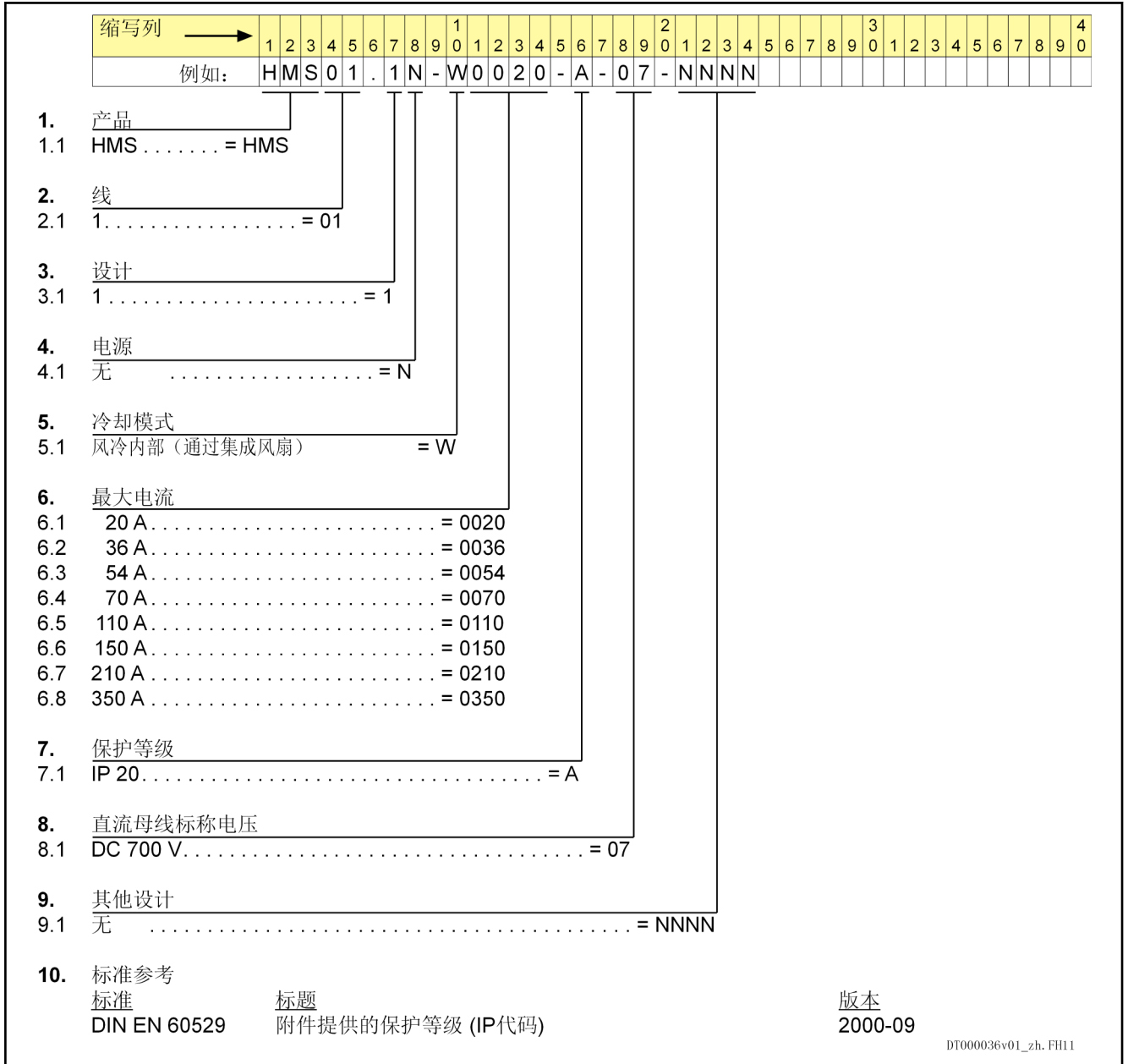
插图 2-1: 类型代码 HMS01
