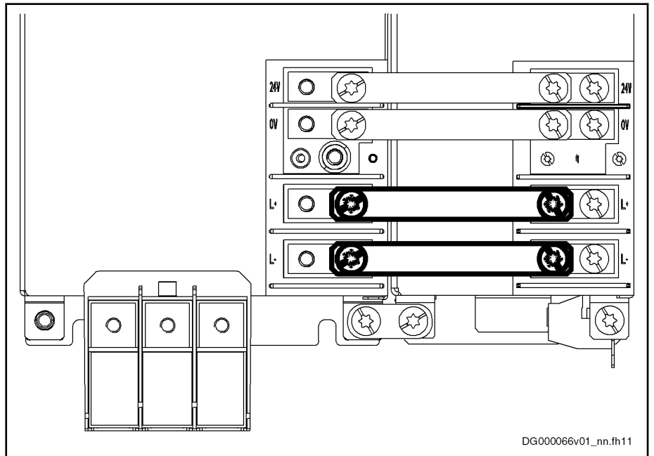
插图 5-6: 带连接排的直流母线连接
